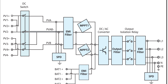
Schaltplan
